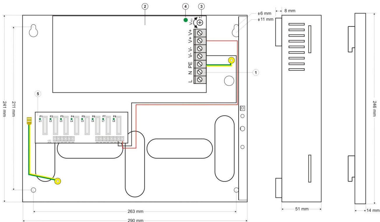
Rys.3. Widok zasilacza.
